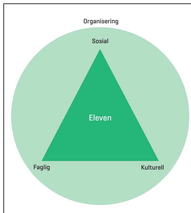
Figur 2.7 Inkluderingsdimensjonene
